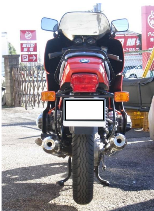
純正と同じ方法で取り付け（右上がり）
